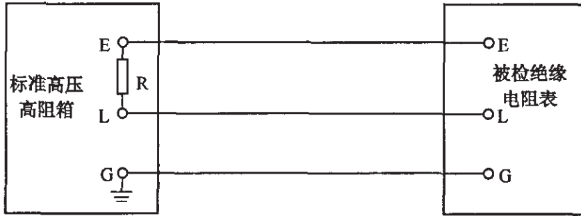
图2 绝缘电阻表基本误差检定接线图
