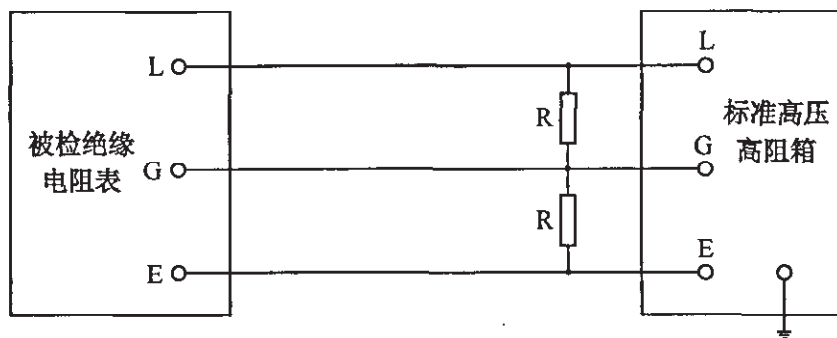
图 4 检查屏蔽装置作用的接线图
