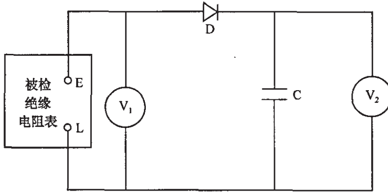
图3 绝缘电阻表端钮电压有效值与峰值测量回路
