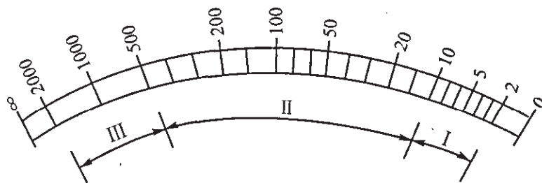
图1 绝缘电阻表量程区段
