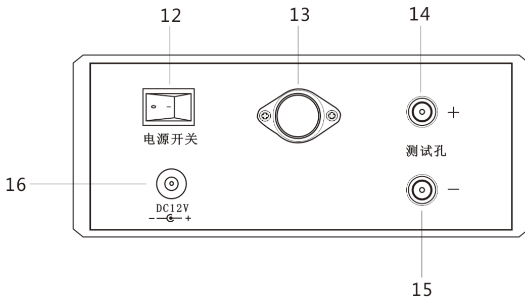
仪器反面面板图
