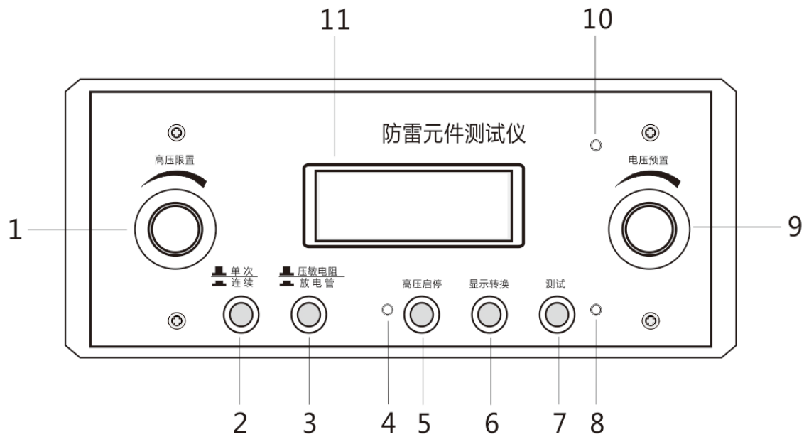
仪器正面面板图
