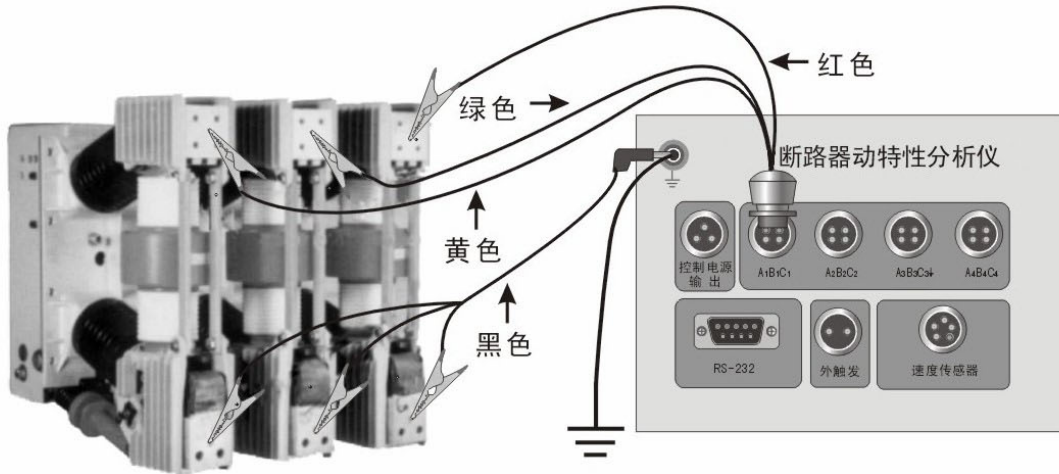
断口接线图（三断口）
